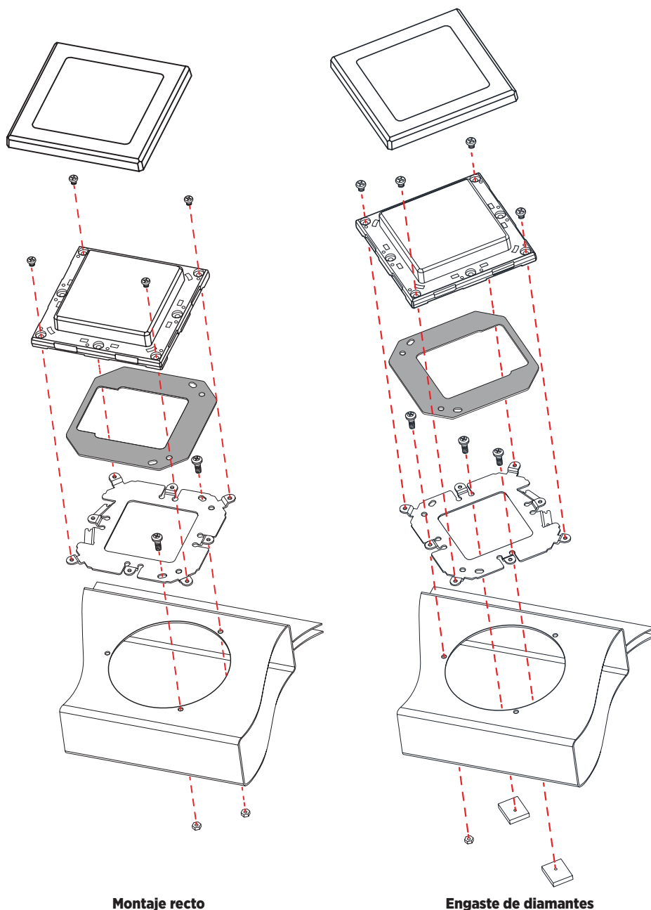
Montaje recto
